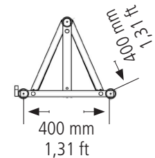
Dettagli colonna verticale Mast section details
